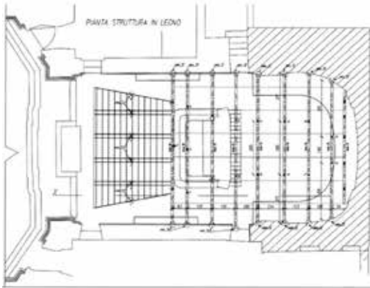
Qui viene presentato lo schema costruttivo della struttura lignea dell'apparato di Travagliato in pianta e in sezione. Disegno dell'ingegner Bettoni
